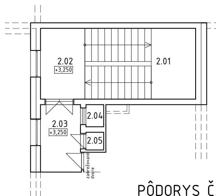
PÔDORYS 2.NP
